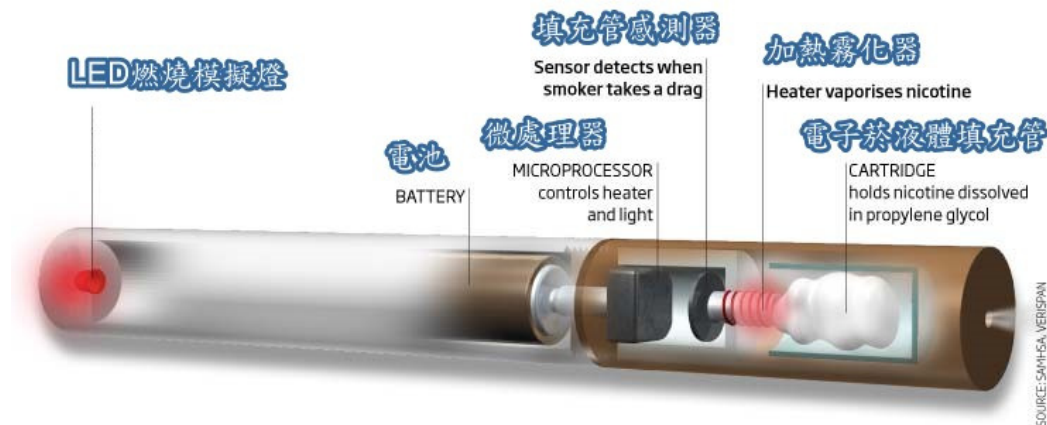
圖 1 電子煙零組件構造圖。(http://www.e-cigarette-direct.com/pages/How-E-Cigs-Work.html)
